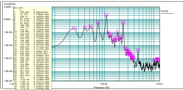
圖 6. 玻璃帷幕振動加速度頻譜圖
