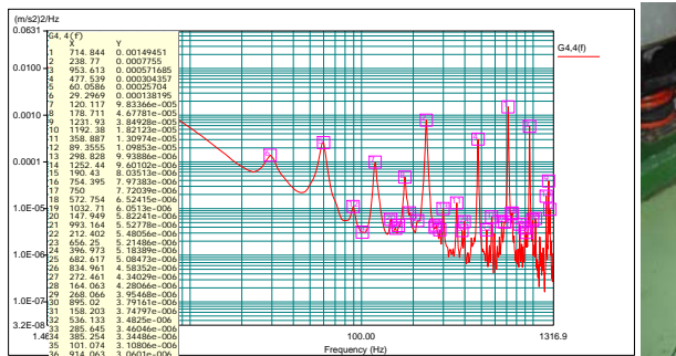
圖 10. 機房機器旁牆面振動加速度頻譜圖
