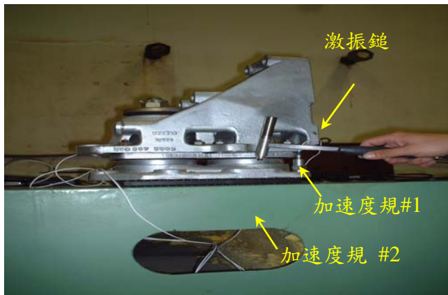
圖 11. 隔振器動性測試平台示意圖
