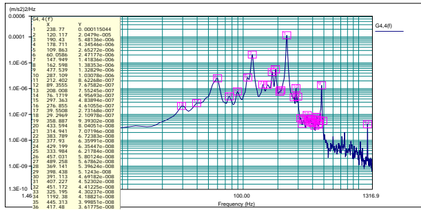
圖 5 辦公室柱面木質板表面振動加速度頻譜圖
