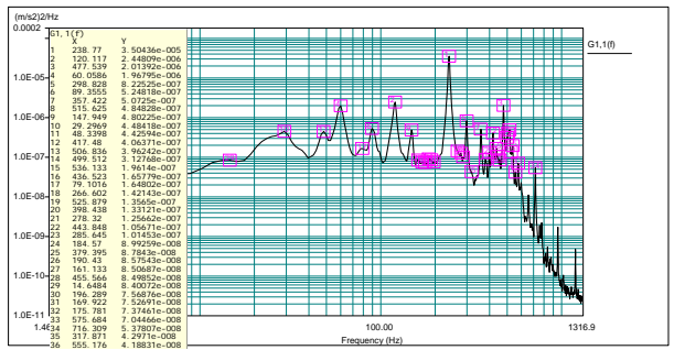
圖 8. 機房樓板振動加速度頻譜圖
