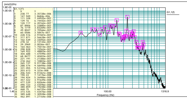
圖 7 辦公室樓板振動加速度頻譜圖
