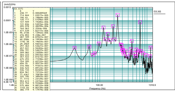
圖 9. 機房鋼柱振動加速度頻譜圖
